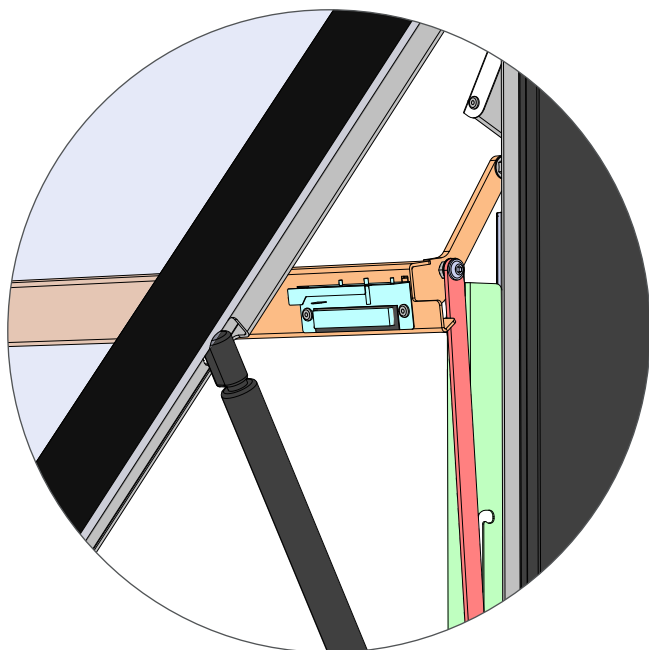
Detail: pohled na hrazdu s upínacími pákovými klipy ve snížené poloze
