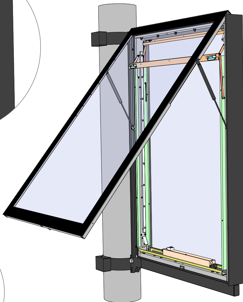
Detail: pohled na hrazdu ve snížené poloze
